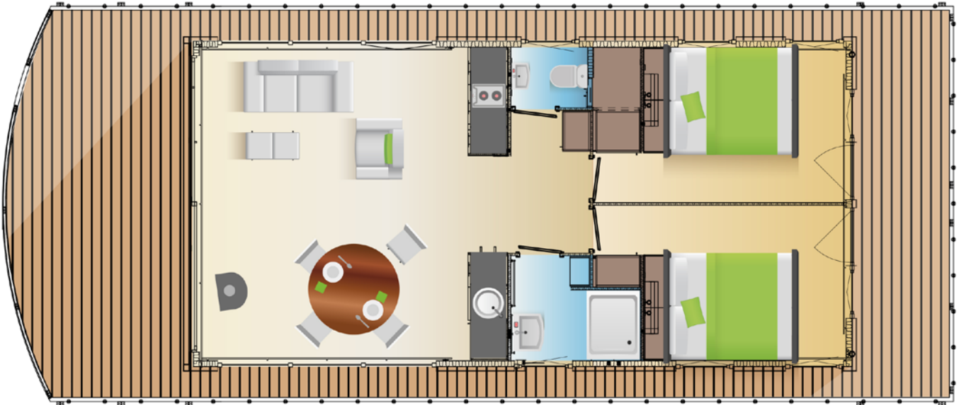
Erdgeschoss - Variante mit Kamin
