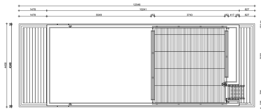
GRUNDRISS OBERDECK
