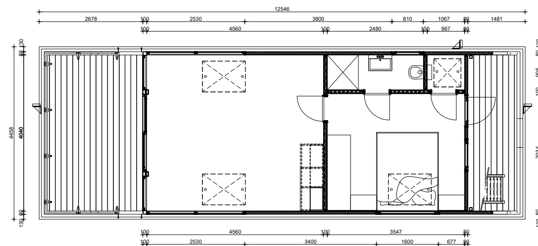
GRUNDRISS HAUS
