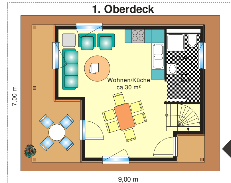
Grundriss Ferienhaus Typ „Ostsee“ mit ca. 70 qm Wohn / Nutzfläche
