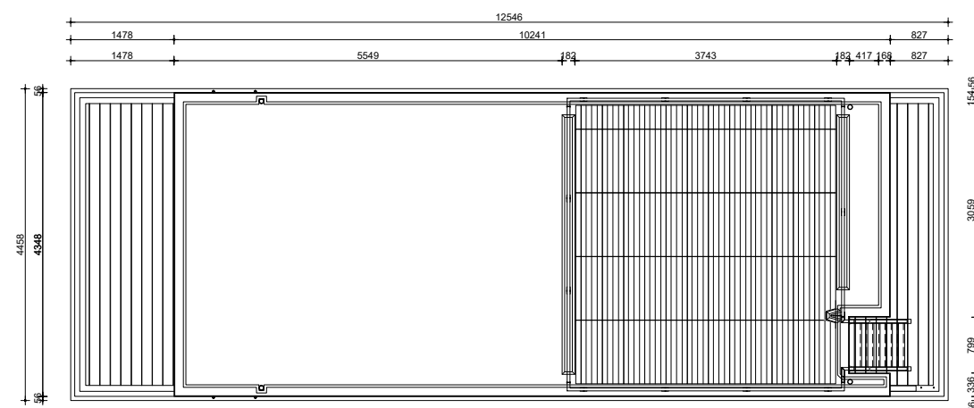
GRUNDRISS OBERDECK
