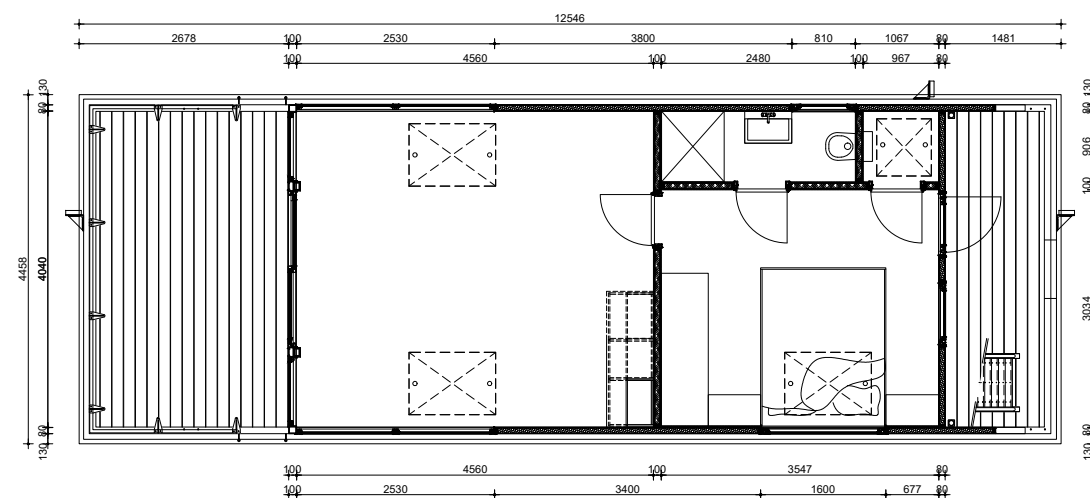
GRUNDRISS HAUS
